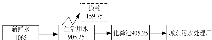
图 2-1 项目水平衡图 (t/a)
