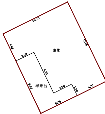
第2层平面图
