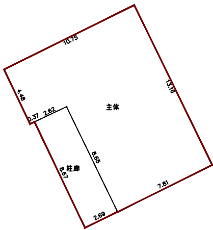
第1层平面图
