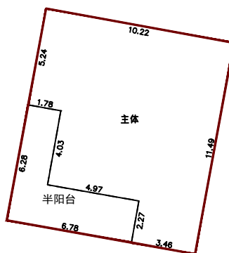
第2层平面图
