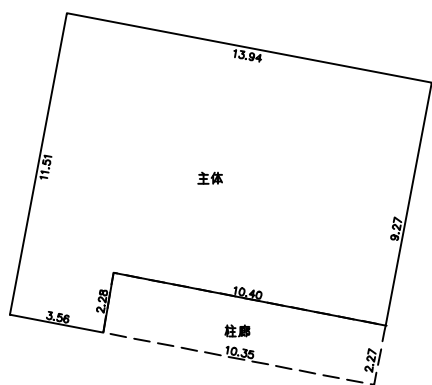
第1层平面图
