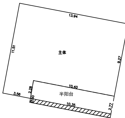
第2层平面图
