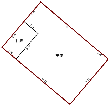
第1层平面图
