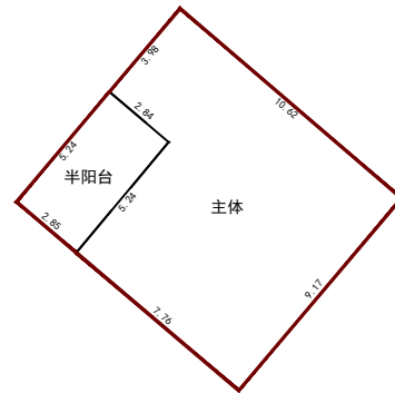
第2层平面图
