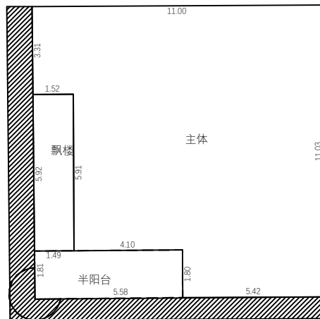
3层平面图
