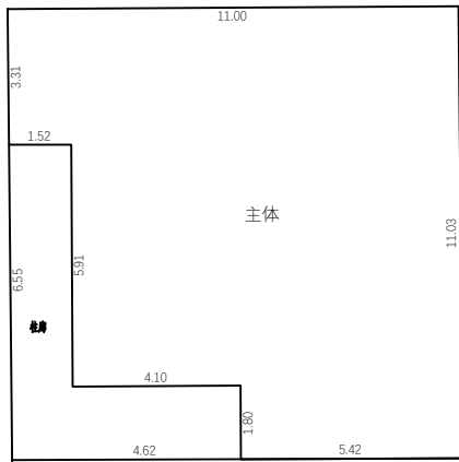
1层平面图
