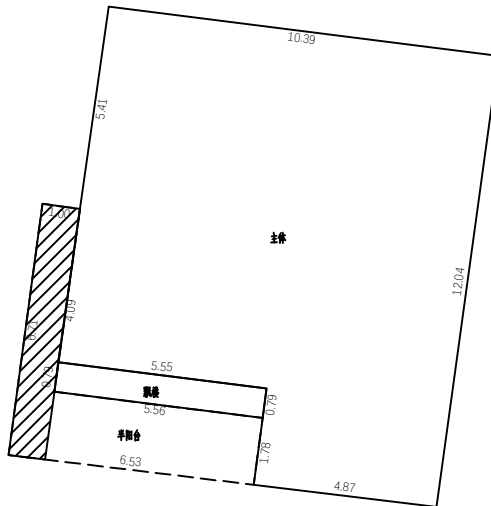
3层平面图
