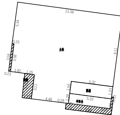
2层平面图
