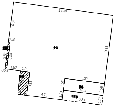
3层平面图
