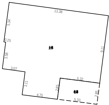
1层平面图
