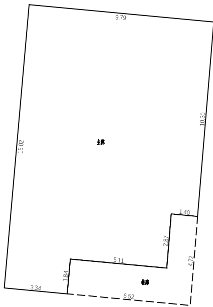
1层平面图
