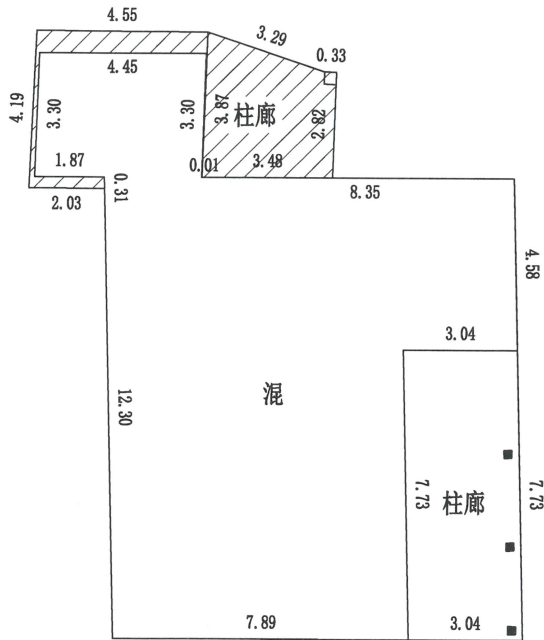
第一层平面图
