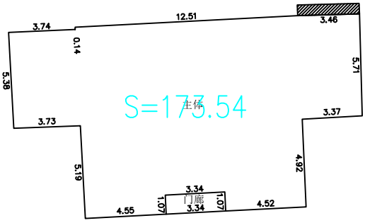
1层平面图
